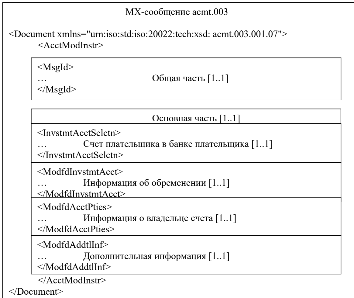
Рисунок 1 – Структура МХ-сообщения acmt.003
